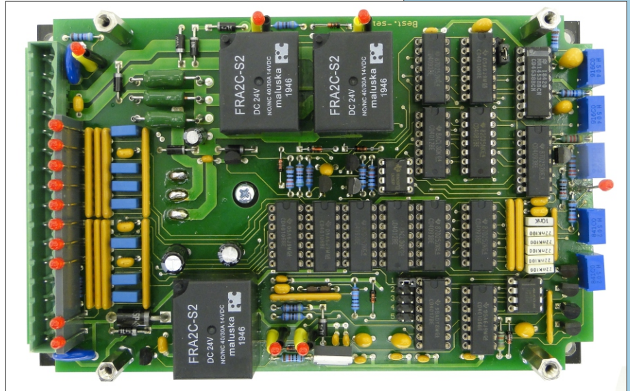
Leiterplatte „offen“
