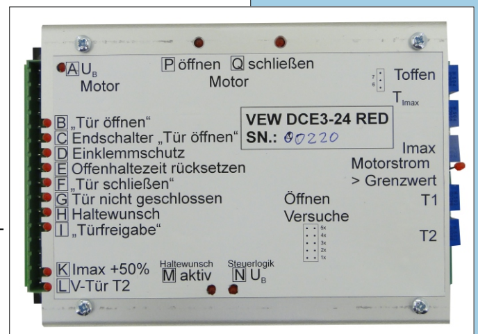
Baugruppe mit Abdeckung
