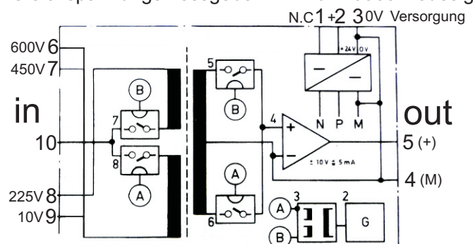
Gleichspannungsmessgeber VEW 6KA9905 Redesign
