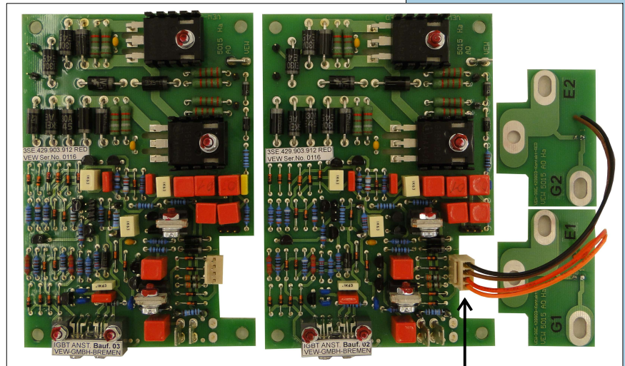
steckbare Verbindung zu den IGBTs
