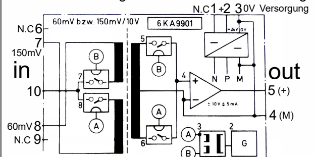
Gleichstrommessgeber VEW 6KA9901 Redesign
